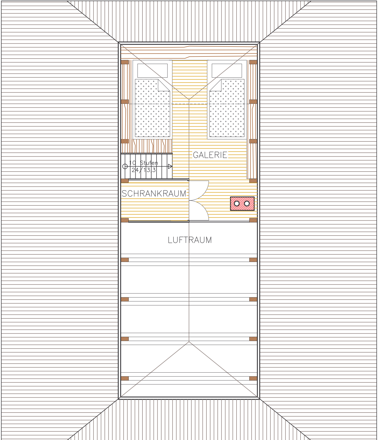
GALERIE 1:50 Wohnnutzfläche 14,90 m 2
